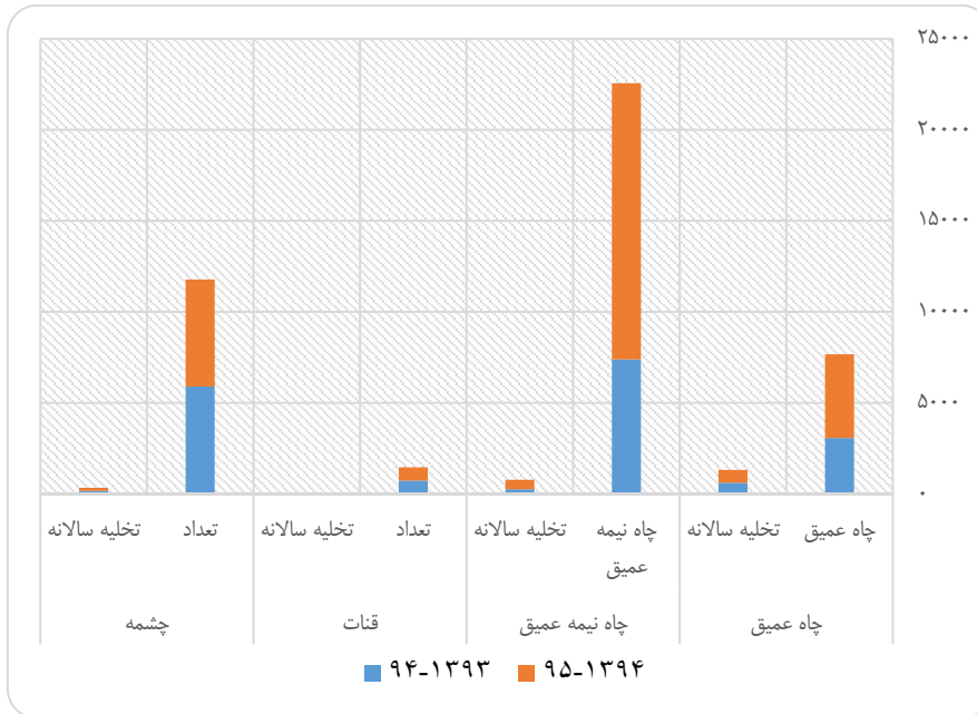
نمودار ۳۲- مقدار تخلیه سالانه آب استان از منابع آب های زیرزمینی در سال آبی ۹۵-۱۳۹۴
