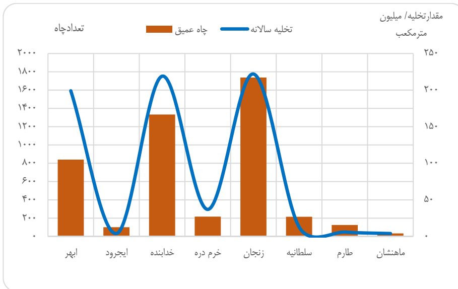
نمودار ۳۳- تعداد و مقدار تخلیه آب زیرزمینی شهرستان ها از طریق چاه عمیق در سال آبی ۹۵-۱۳۹۴
