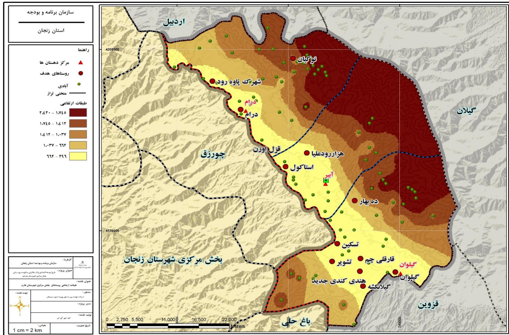
نقشه ۱۲: طبقات ارتفاعی بخش مرکزی شهرستان طارم
