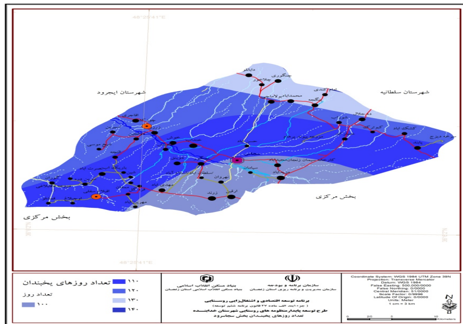
شکل ۱۳. تعداد روزهای یخبندان بخش سجاسرود شهرستان خدابنده
