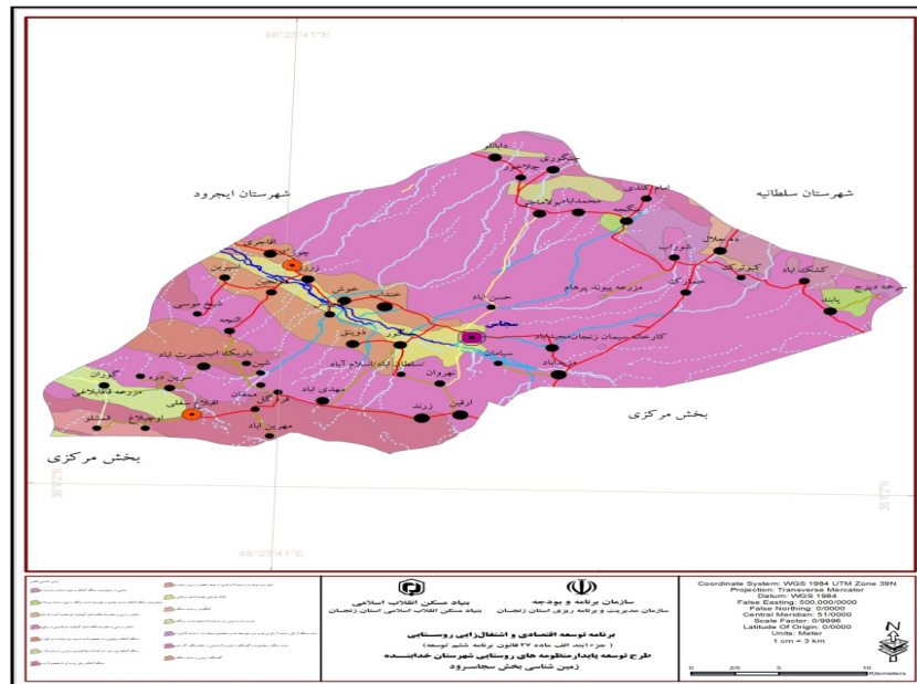
شکل ۷. نقشه‌ی زمین‌شناسی بخش سجاسرود شهرستان خدابنده
