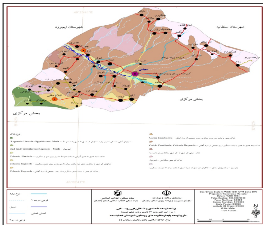
شکل ۸. نوع خاک بخش سجا سرود شهرستان خداآبند
