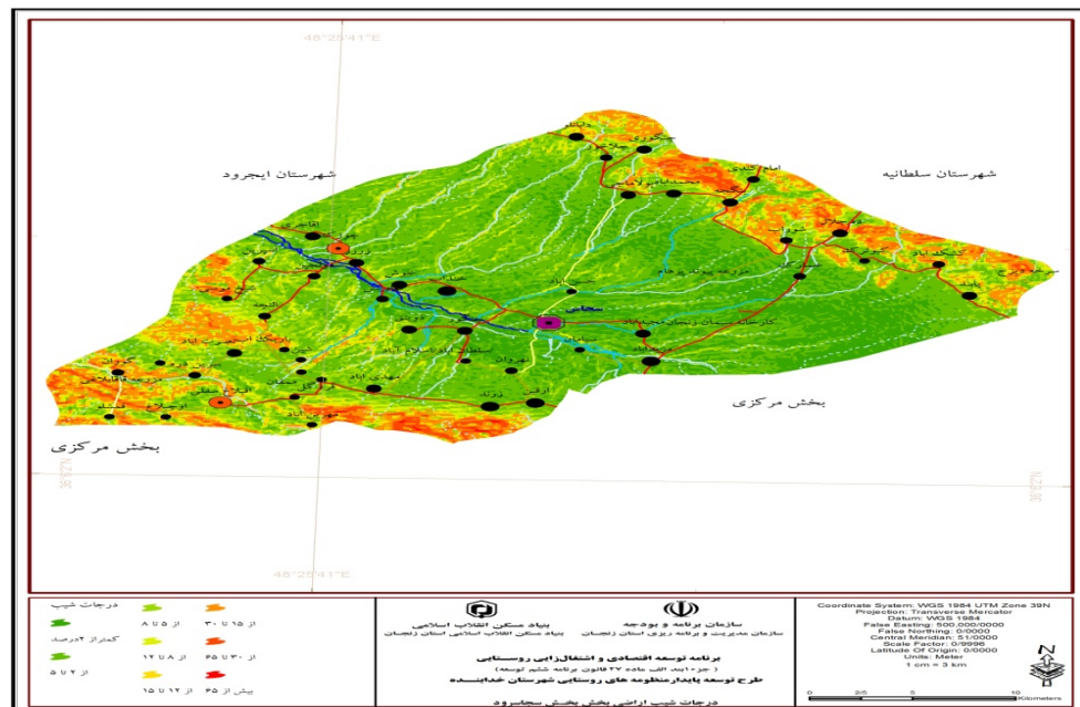
شکل ۱۰. درجات شیب بخش سjasرود شهرستان خداآبنده
