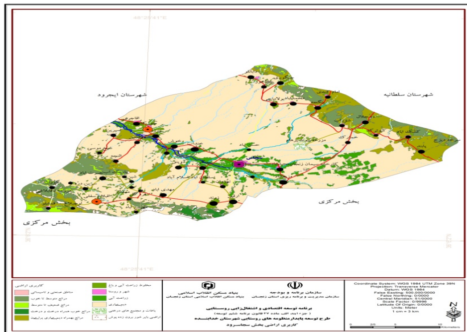
شکل ۱۲. کاربری اراضی بخش سجاسرود شهرستان خدابنده
