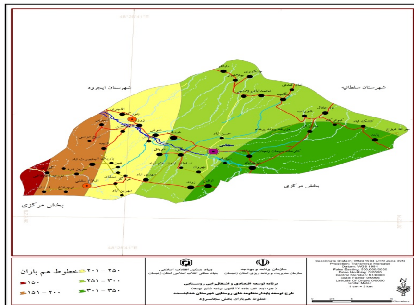
شکل ۱۴. میزان بارندگی بخش سجاسرود شهرستان خدابنده
