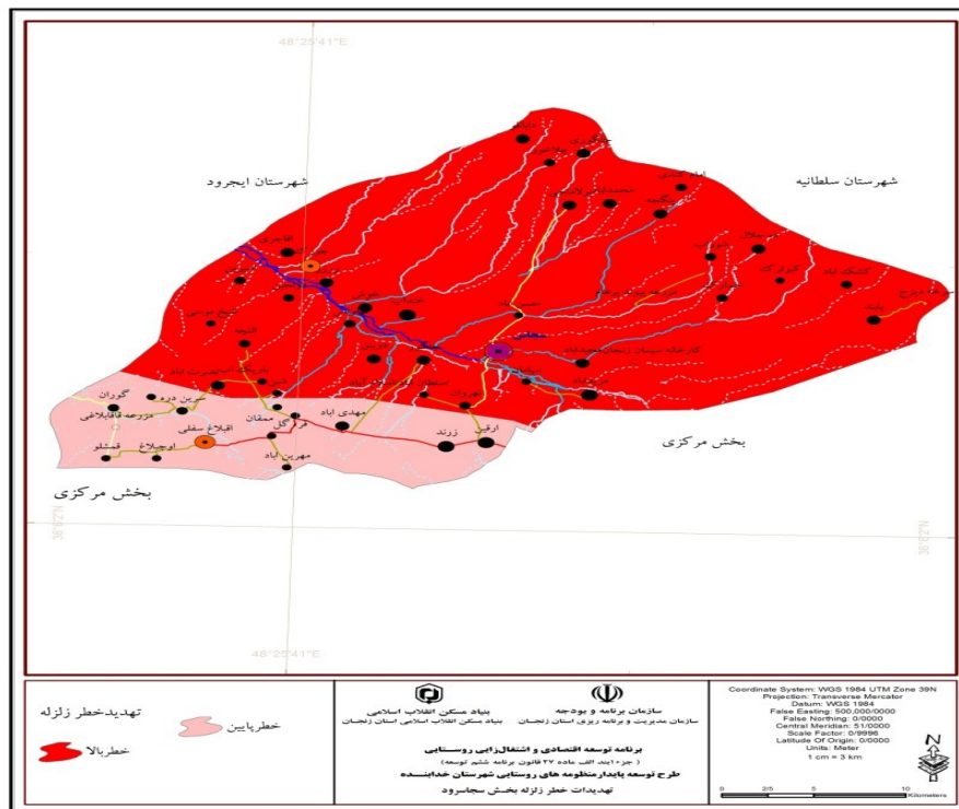
شکل ۱۸. رانش و لغزش زمین در بخش سjasرود شهرستان خدابنده
