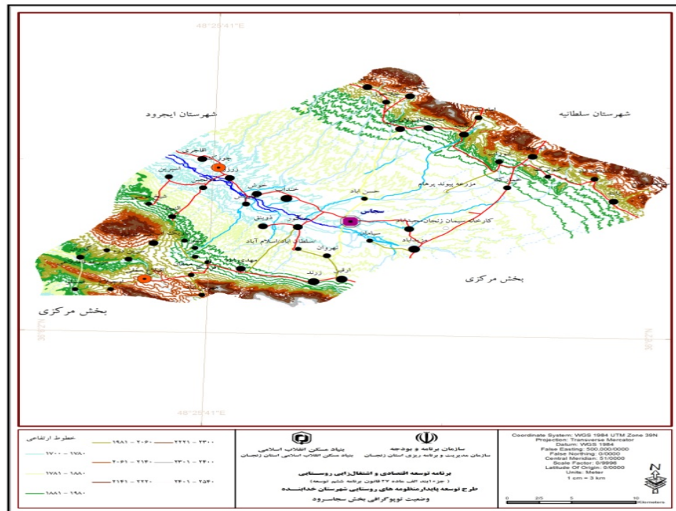
شکل ۹. توپوگرافی بخش سجاسرود شهرستان خدابنده
