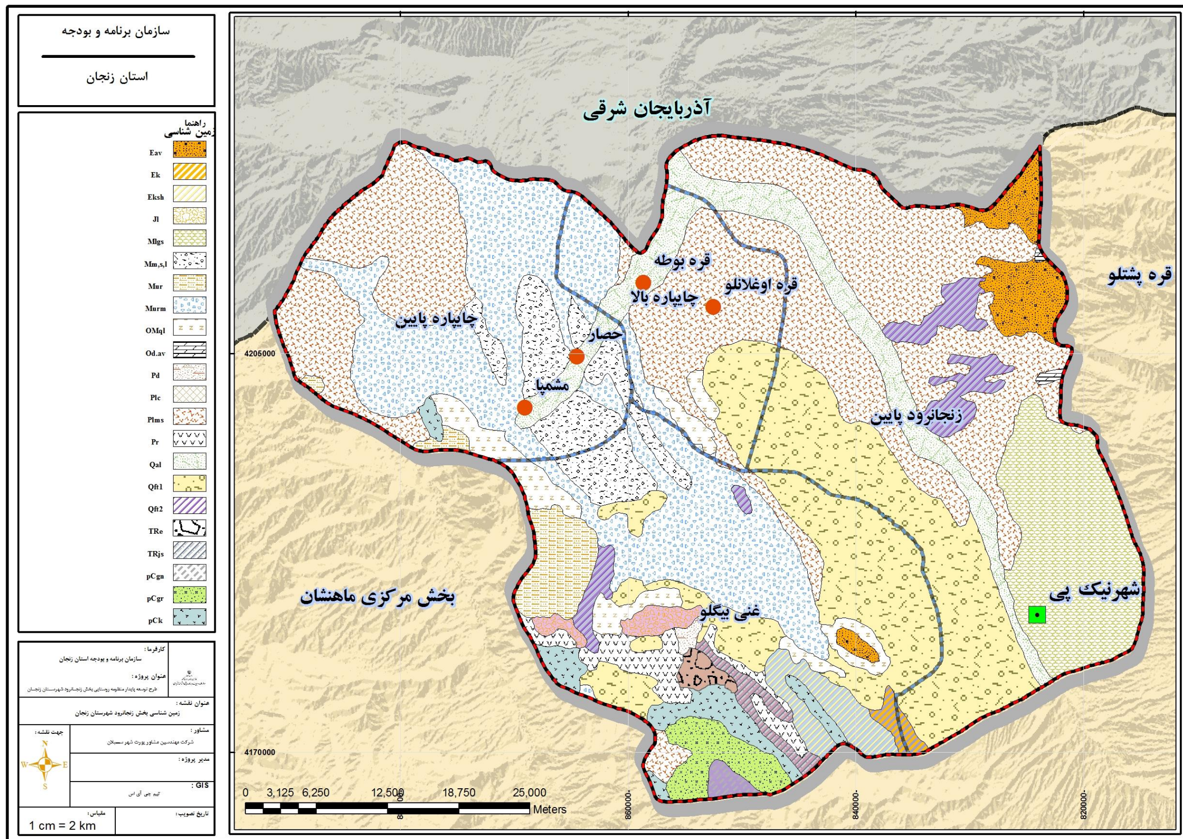
نقشه ۱۰: زمین شناسی بخش زنجانرود شهرستان زنجان
